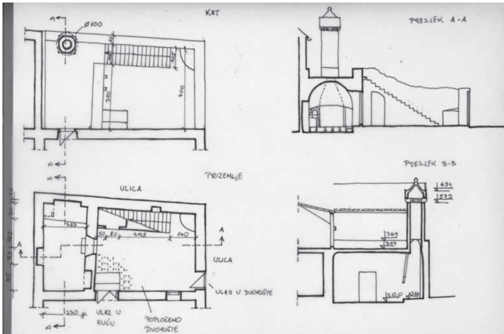
Sl. 3.08 Tlocrt kominata u Dvornjoj Luci
